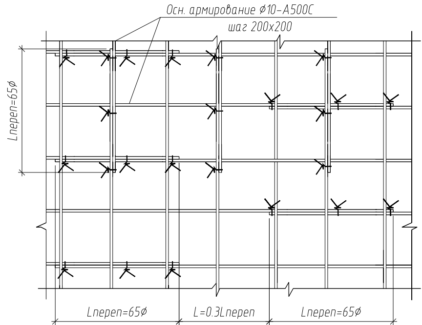
Узел стыковки арматуры по длине внахлест
