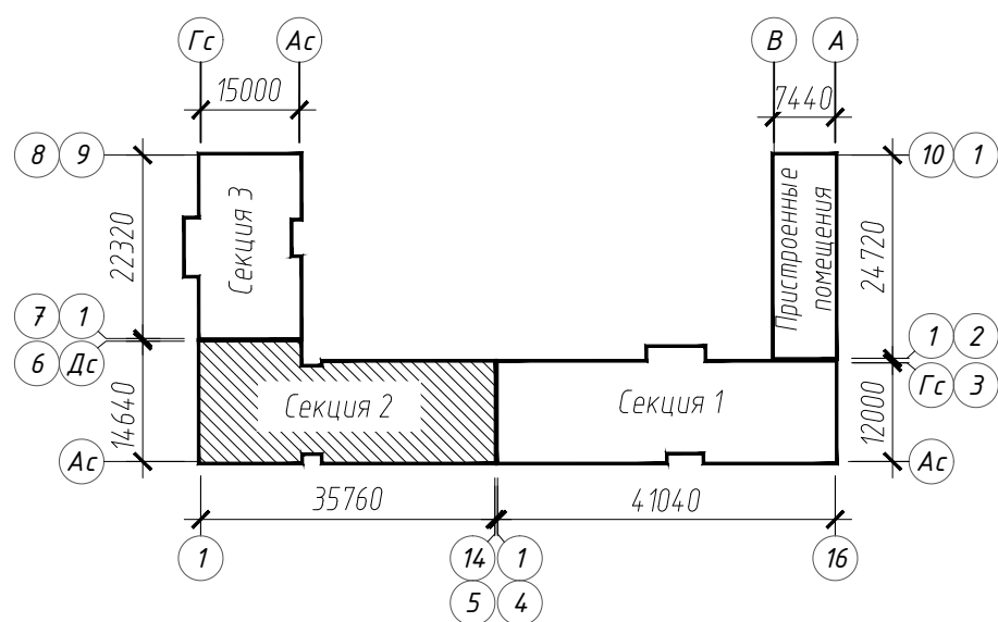
Схема блочировки
