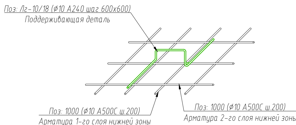
Фрагмент установки фиксирующих элементов поз: Лг-10/18
