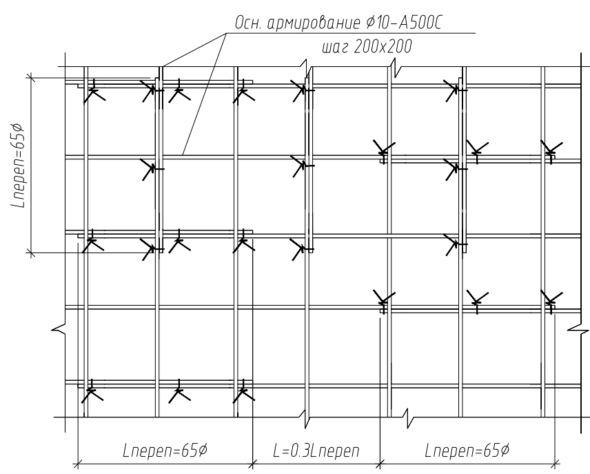
Узел стыковки арматуры по длине внахлест
